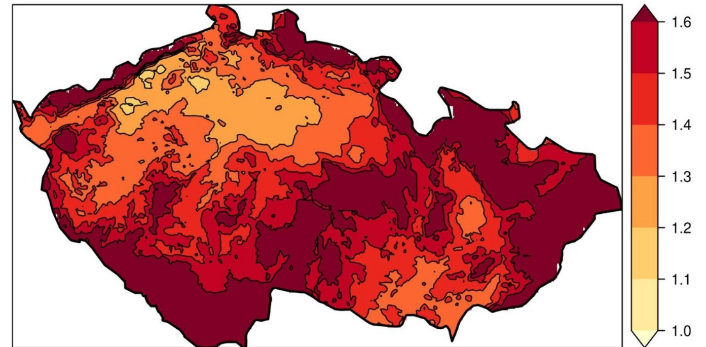
Změny Rfaktoru (2100 | RCP 8.5)
