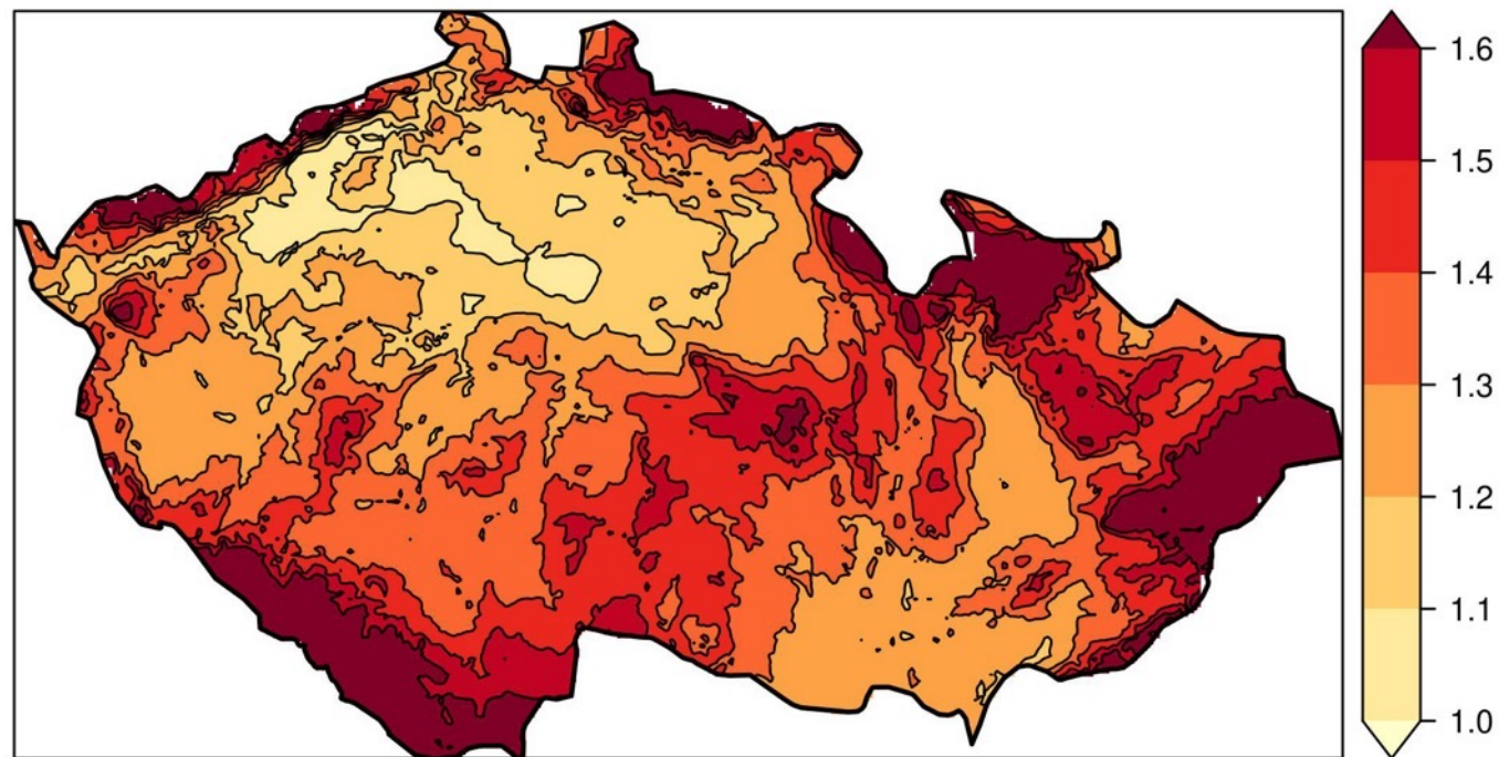
Změny Rfaktoru (2050 | RCP 8.5 = 2100 | RCP 4.5)
